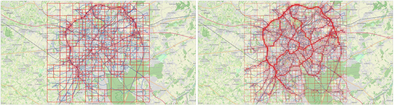
Figura 3.1: Grilla multiresolución sobre datos de Bruselas obtenidos mediante el generador BerlinMOD. Cada celda contiene como máximo 10.000 (izquierda) y 1.000 (derecha) instantes durante todo el período de simulación (cuatro días en este caso). A la izquierda, podemos ver la alta densidad de tráfico en el anillo alrededor de Bruselas, mientras que a la derecha podemos ver otros ejes principales de la ciudad.
