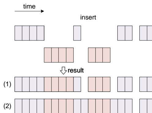
Figura 6.1: Operación de inserción para valores temporales.
