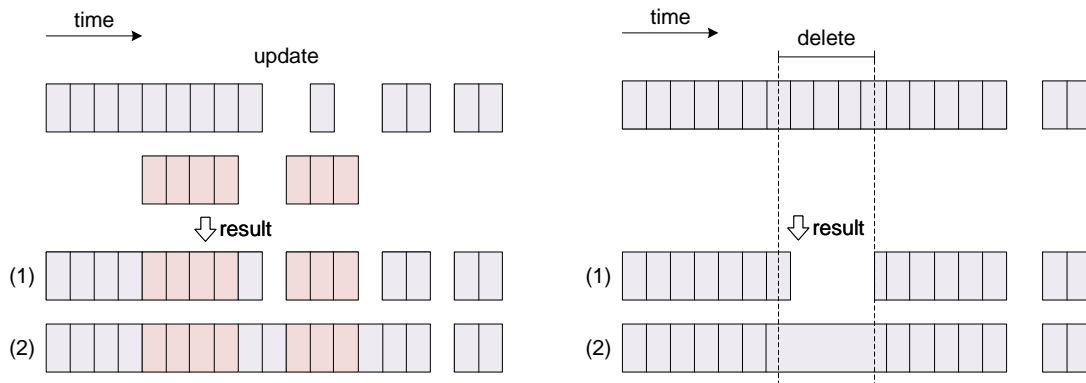
Figura 6.2: Operaciones de actualización y supresión para valores temporales.
