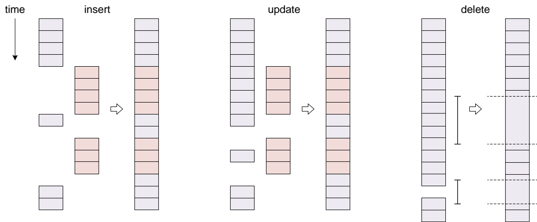
Figura 6.3: Operaciones de modificación para tablas temporales en SQL.
